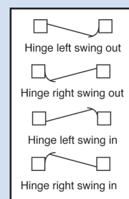
Single hinge door
